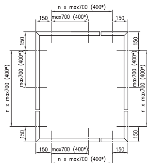
OŚCIEŻNICA OKNA ROZMIESzcZENIE KOTEW/DYBLI RAMA OKIENNA
